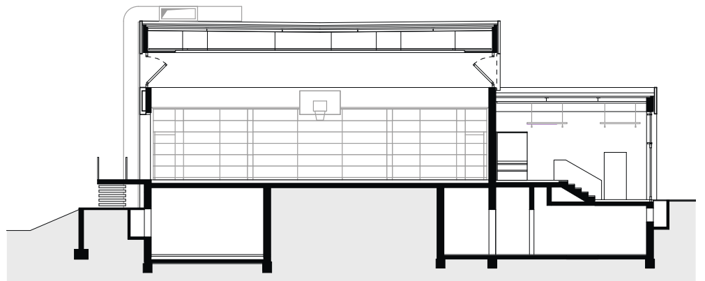
Querschnitt durch Sporthalle and Gastronomie
